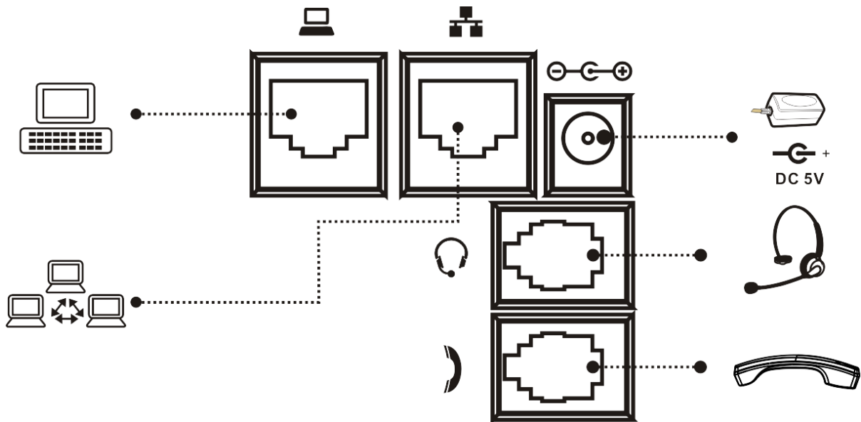
그림 3 - 장비 연결
