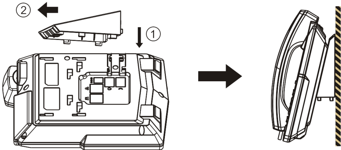
그림 2 - 벽면 설치
